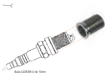
REF: 105205 TORRE BUJIA CUATRO TIEMPOS Rosca: Exterior 1/2, Interior M10
