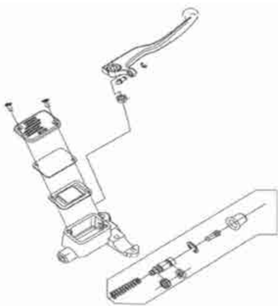
KIT DE REPARACIÓN BOMBA DE FRENO
